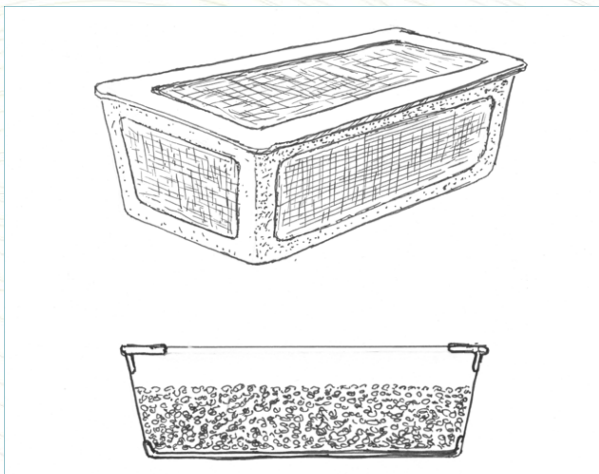
Obr. 48. Schéma odchovné klíčky. Klíčka je vyrobena z plastové dózy s vyříznutými otvory překrytými síťovinou (nahore) a vyplněna tříděným hrubým pískem (dole). Kresba: Michal Bílý.
