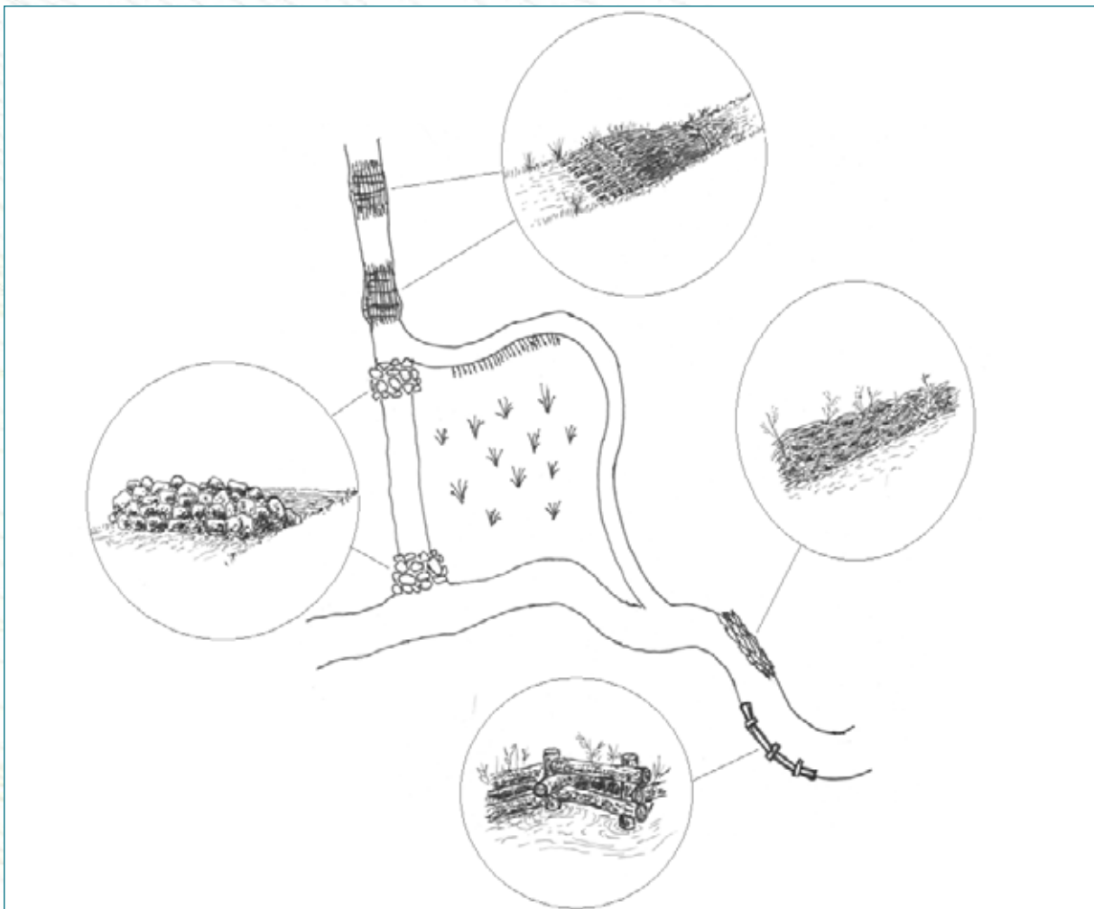
Obr. 149. Příklad kombinovaného opatření stabilizace erozí poškozeného koryta. Vrbo-olšové rošty, kamenné částečně protékané uzávěry a vyvedení vody z erodovaného koryta, hafošterkový oživený válec a srubová oživená konstrukce z vrb. Kresba: Michal Bílý.
