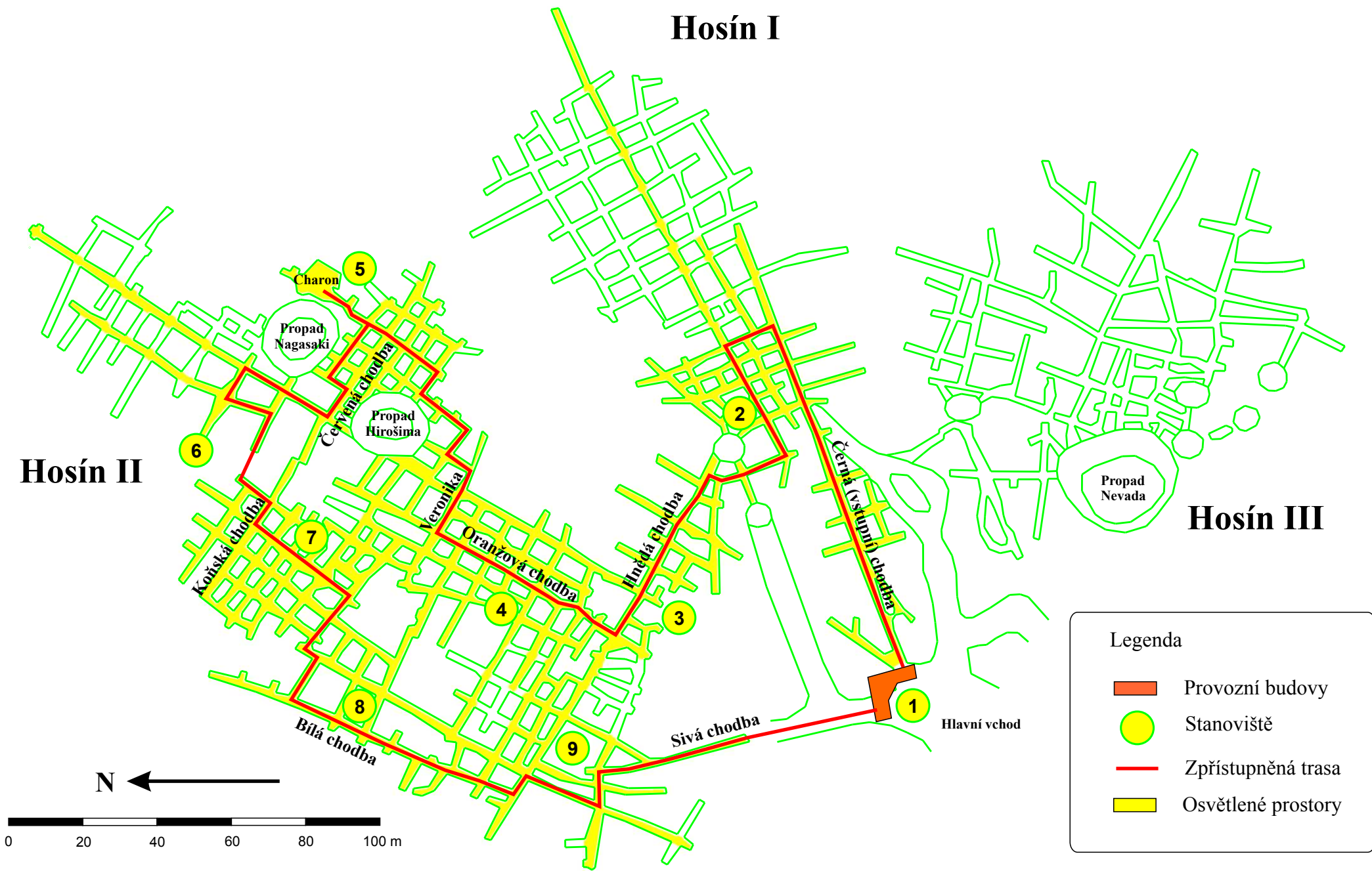
Návrh osvětlení podzemních prostor
